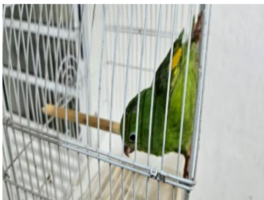
(58490) Periquito-de-encontro-amarelo
